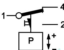
Срабатывание контактов при ручном сбросе низкого давления
