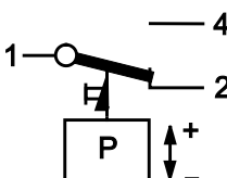
Срабатывание контактов при ручном сбросе высокого давления
