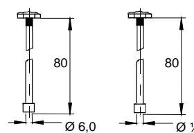
U X 6 мм / 1/4" ODF пайка трубка длиной 80 мм
