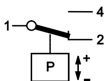
Срабатывание контактов при автоматическом сбросе
