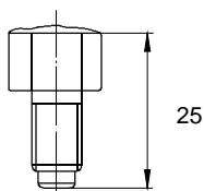
A 7/16" -20 UNF наружная резьба (1/4"SAE)
