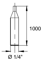
L 1/4" пайка трубка длиной 1 м Замена для R08
