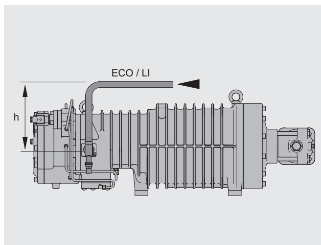
Abb. 4 Rohrführung bei Economiser und Kältemittel-Einspritzung Fig. 4 Piping with Economiser and liquid injection Рис. 4 Трубопровод экономайзера и впрыска жидкости
