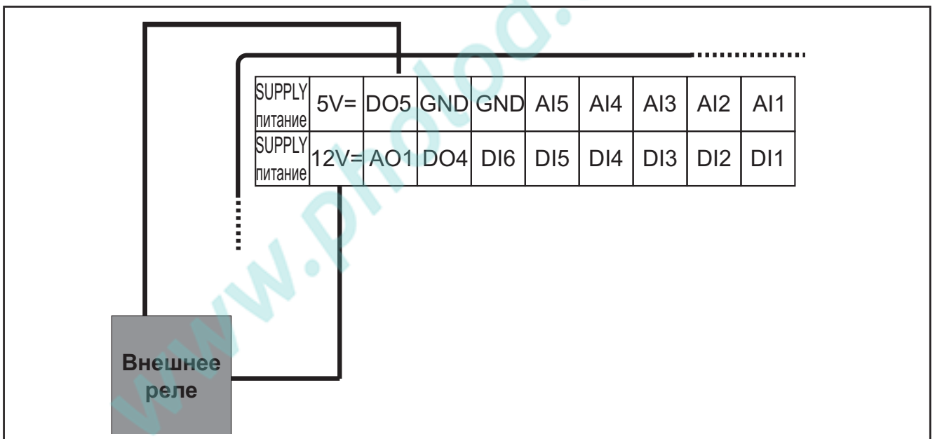
Рис. 25. Пример подключения внешнего реле к выходу DO5 (Открытый коллектор)
