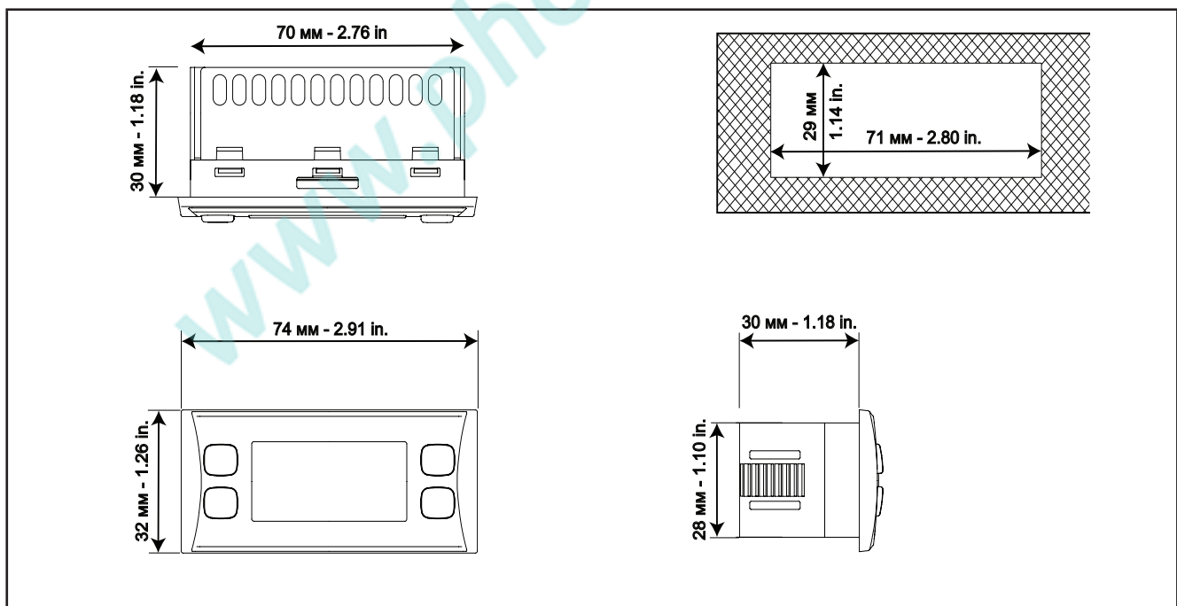
Рис. 29. Размеры внешней клавиатуры SKP 10
