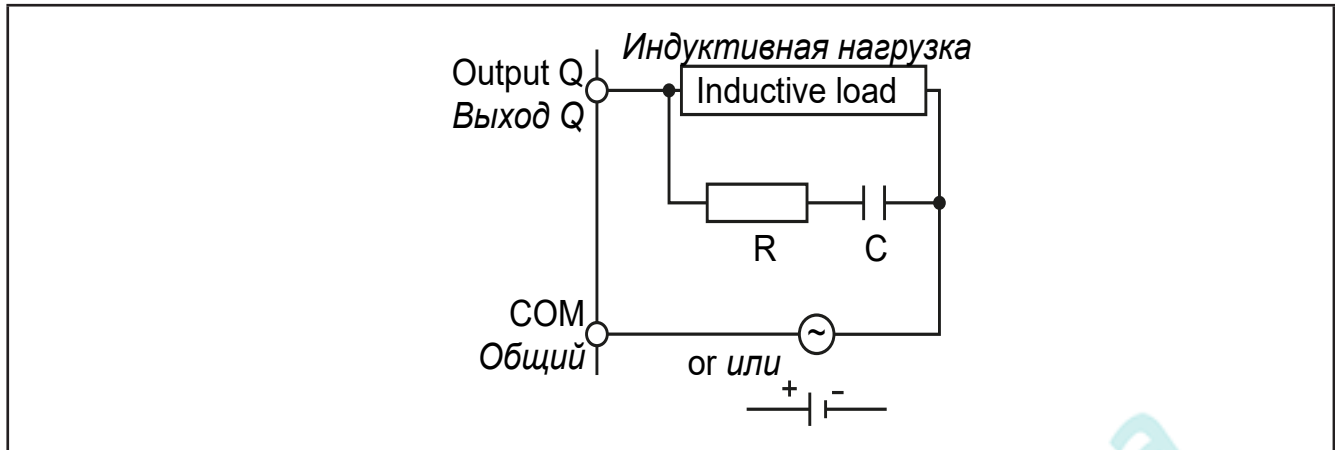
Рис. 12. Защитная цепь типа А
