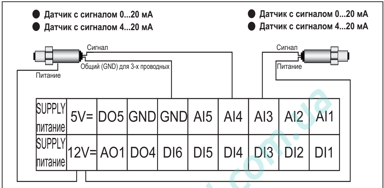
Рис. 18. Подключение датчиков с токовым сигналом
