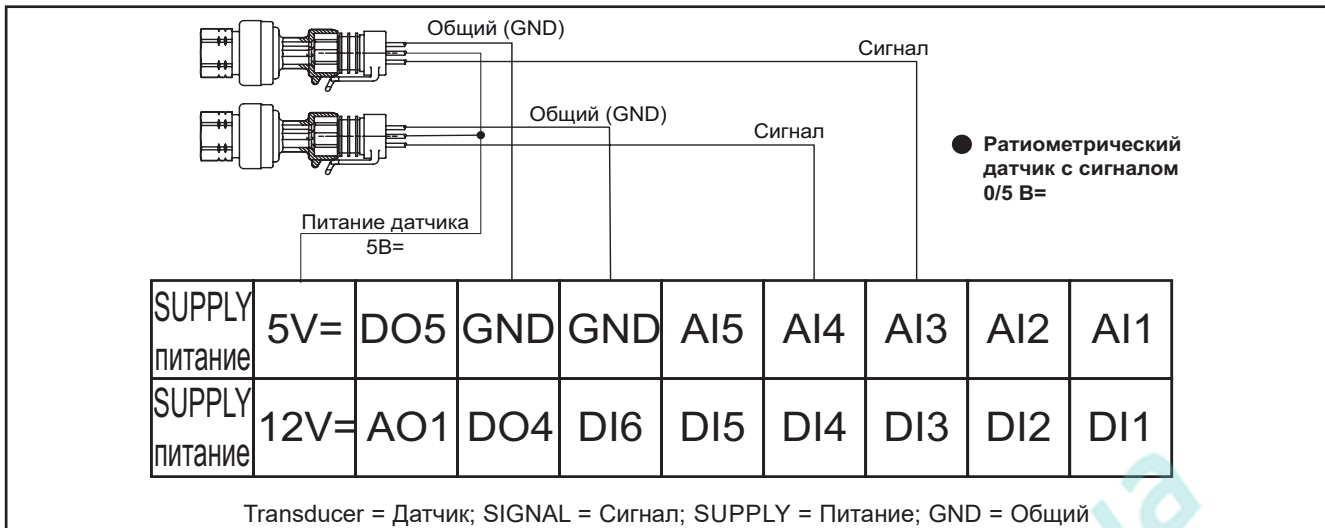
Рис. 20. Подключение ратиометрических датчиков с сигналом 0-5 В
