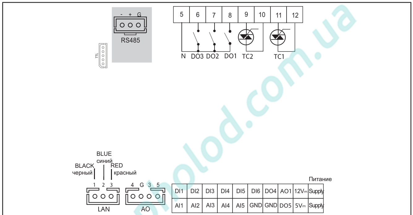
Рис. 16. EWCM 436D PRO /A-CR11
