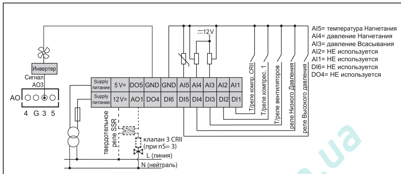
Рис. 26. Стандартное использование цифровых и аналоговых входов
