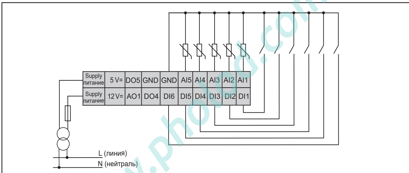
Рис. 21. Пример подключения датчиков температуры и цифровых входов
