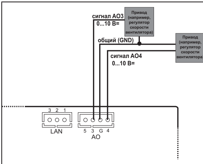
Рис. 23. Пример подключения к выходам AO3 и AO4 модулей регулирования скорости с сигналом 0-10 В
