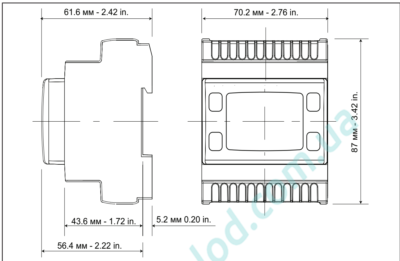
Рис. 28. Размеры контроллера EWCM 436D PRO /A-CR11
