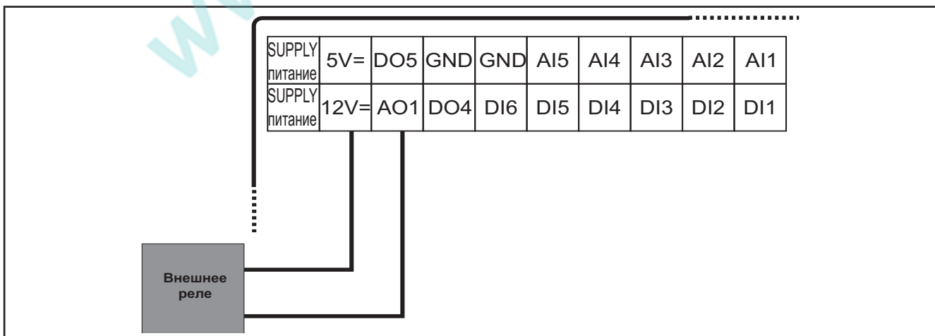
Рис. 22. Пример подключения внешнего реле на выход AO1 (Открытый коллектор)
