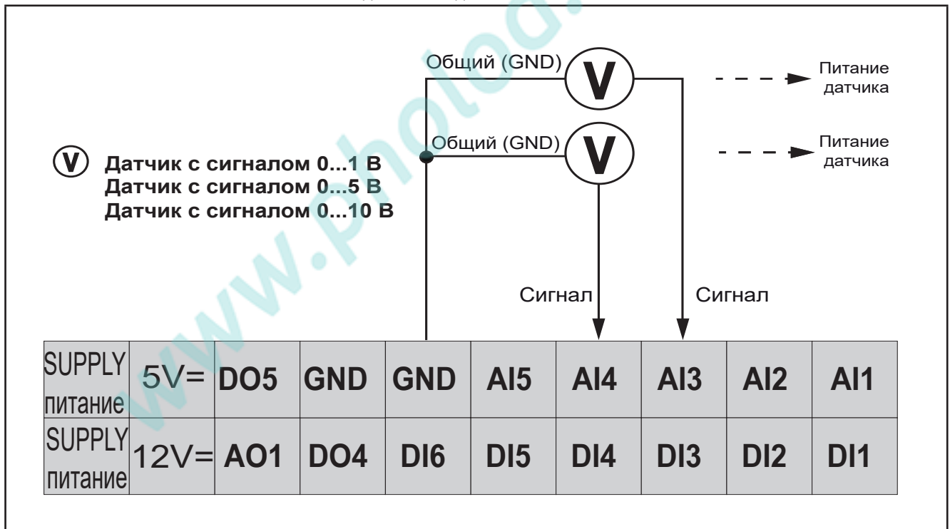
Рис. 19. Подключение датчиков с сигналом напряжения
