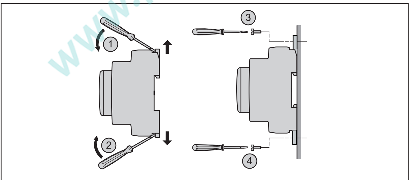
Рис. 8. Установка на панель
