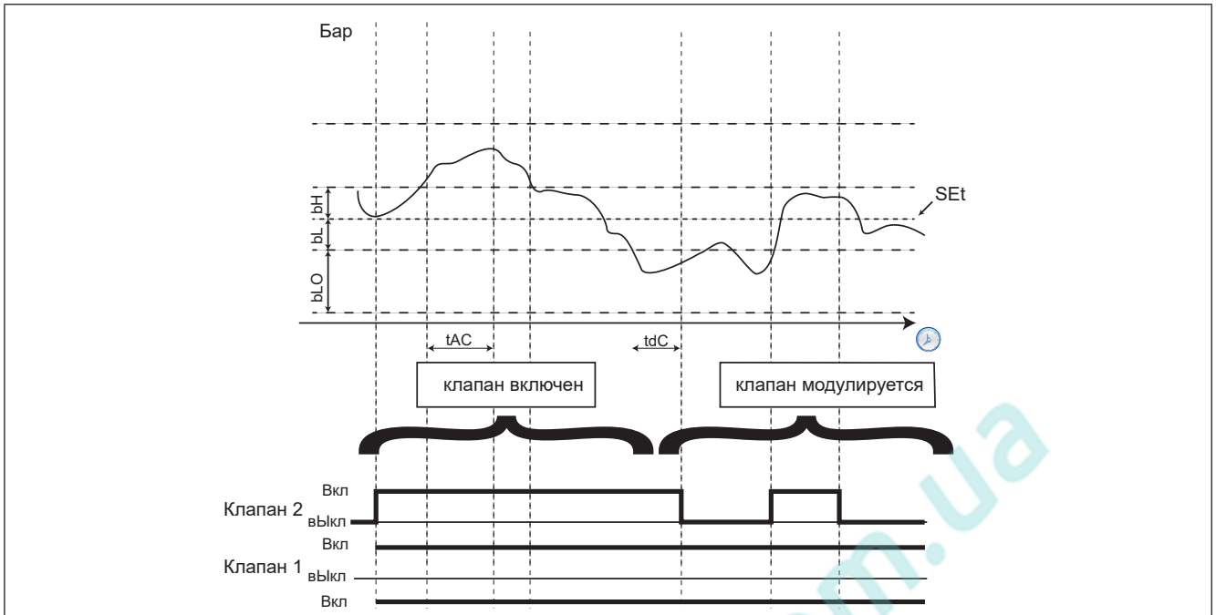
Рис. 35. Отключение клапана
