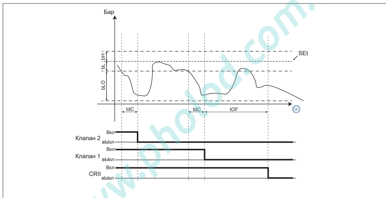
Рис. 36. Выключение компрессора CR11
