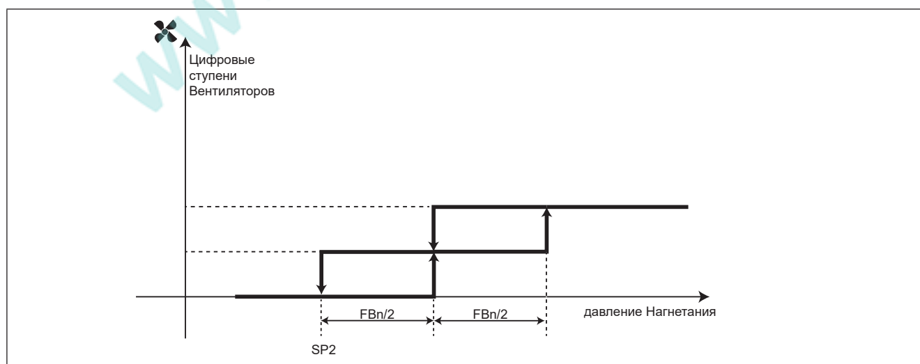
Рис. 37. Управление цифровыми вентиляторами
