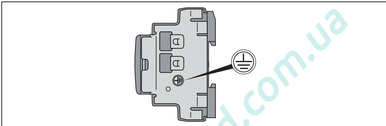
Рис. 17. Заземление EWCM 436D PRO /A-CR11
