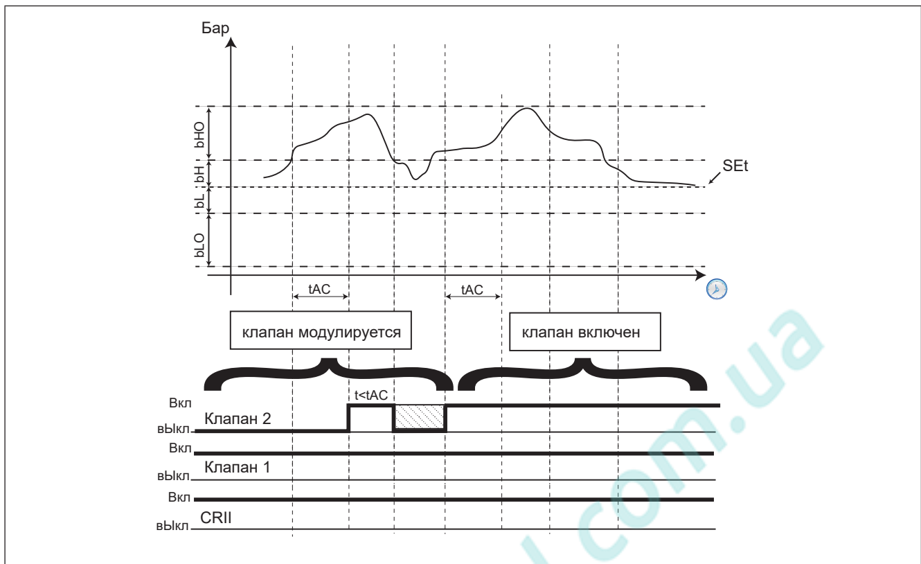
Рис. 34. Перевод клапана 2 из режима регулирования в открытое состояние
