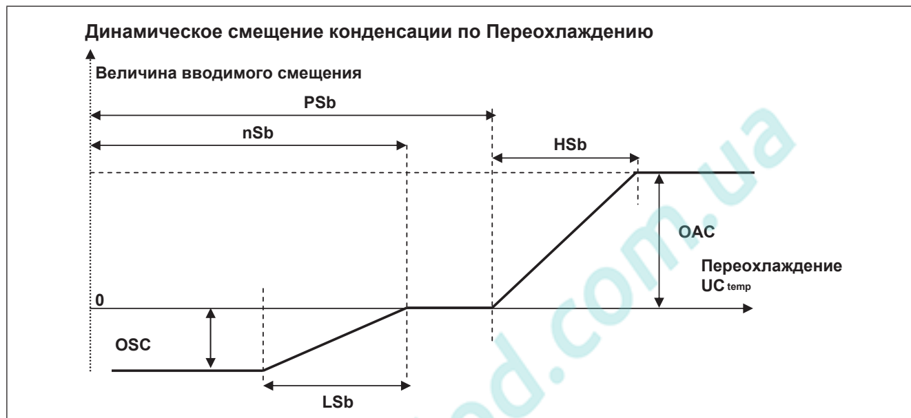
Рис. 39. Плавающая (динамическая) конденсация по переохлаждению
