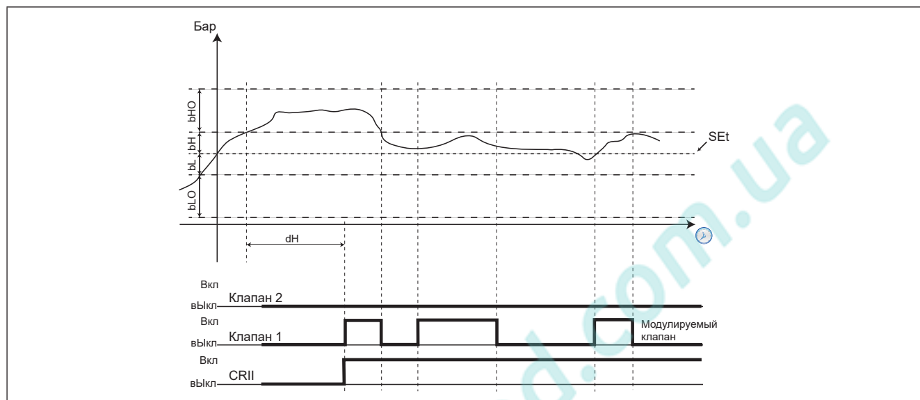
Рис. 32. Запуск компрессора CRII
