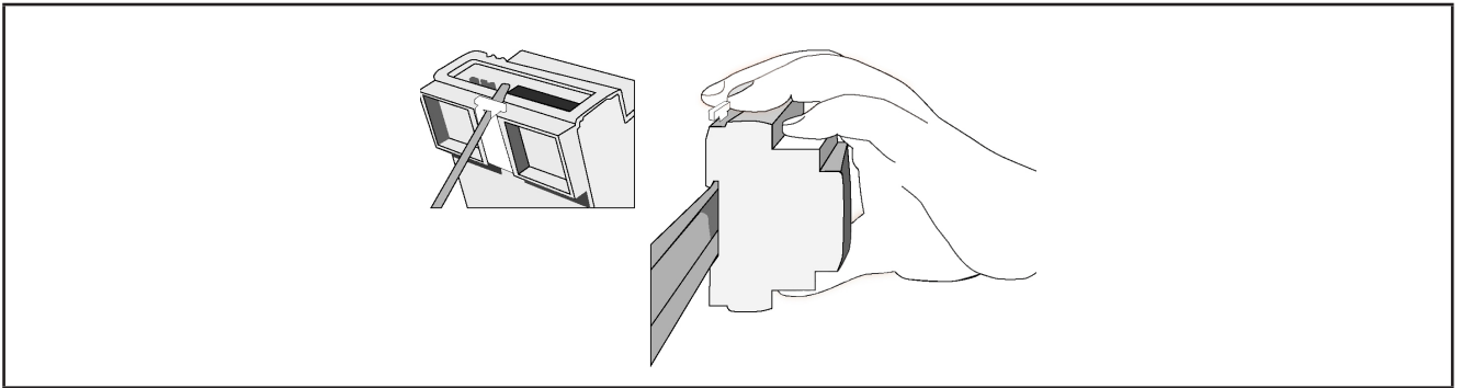
Рис. 6. Установка на DIN рейку – вид ¾
