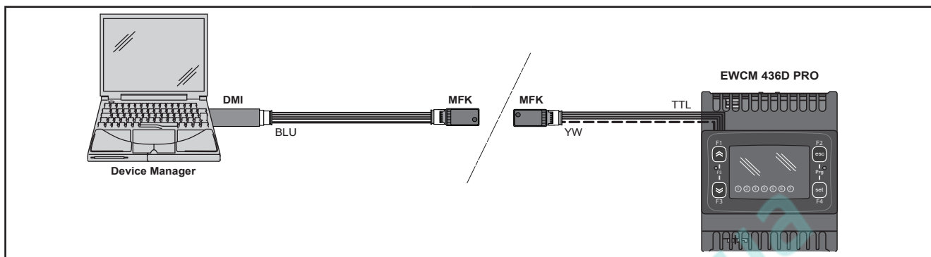
Рис. 41. Подключение MFK 100 к ПК с программой Device Manager и контроллеру
