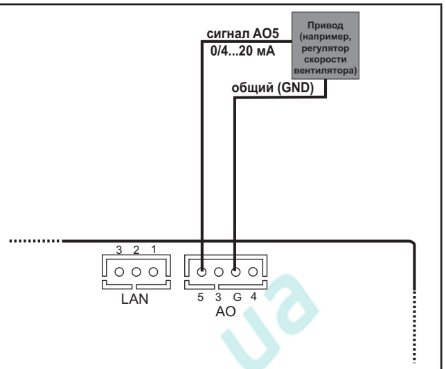
Рис. 24. Пример подключения к выходу AO5 модуля регулирования скорости с токовым сигналом 0/4...20 мА
