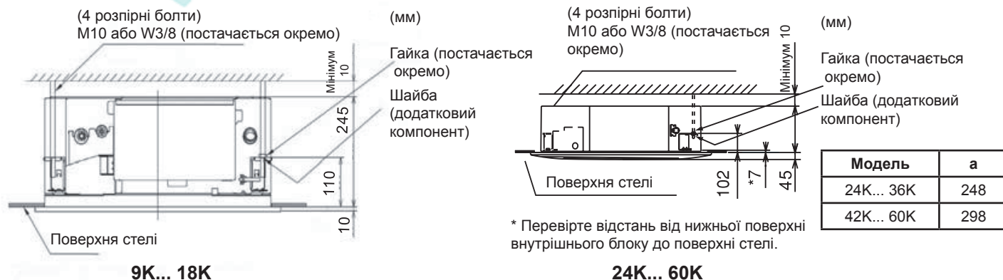
Рис. 3.5. Монтажні положення
