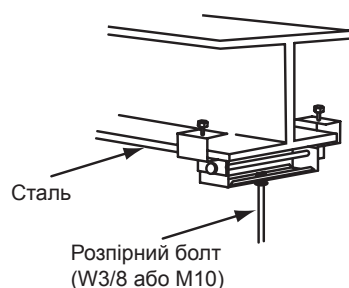
Рис. 3.4. Встановлення розпірних болтів
