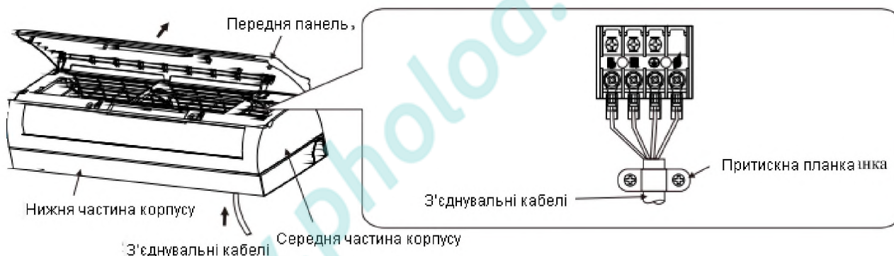
Схема електричного підключення – постійний струм
