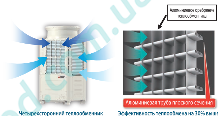
Четырехсторонний теплообменник
