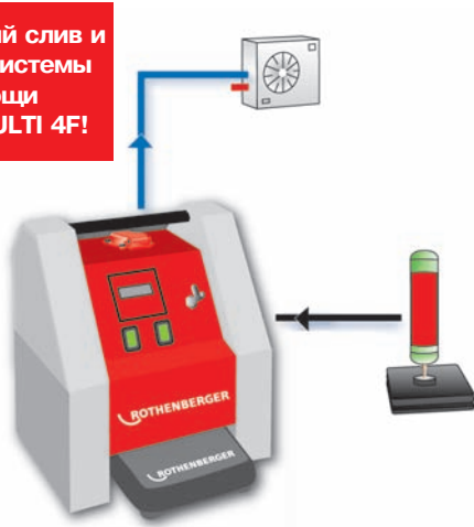
Применение ROKLIMA® MULTI 4F (слив и заполнение).
